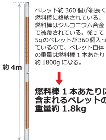
燃料棒
