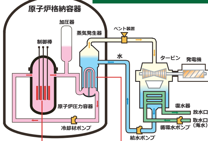
図3 蒸気発生器
