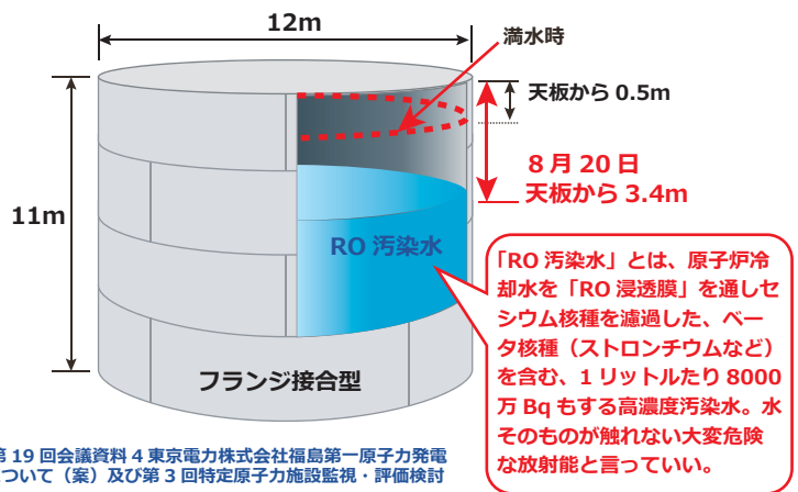
図2 汚染水タンクの詳細
