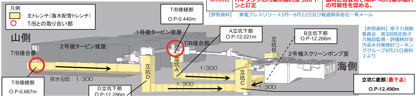
図6 2号機主トレンチ及び立坑立体図
