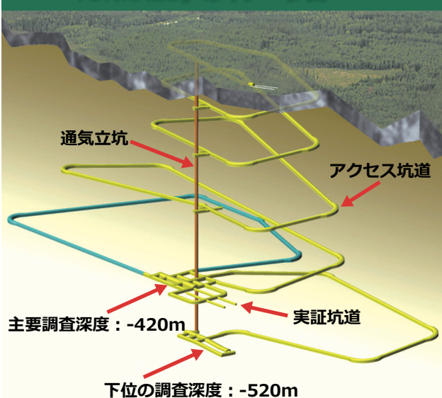
図1 フィンランドの核廃棄物最終処分場「ONKALO」のイメージ図
