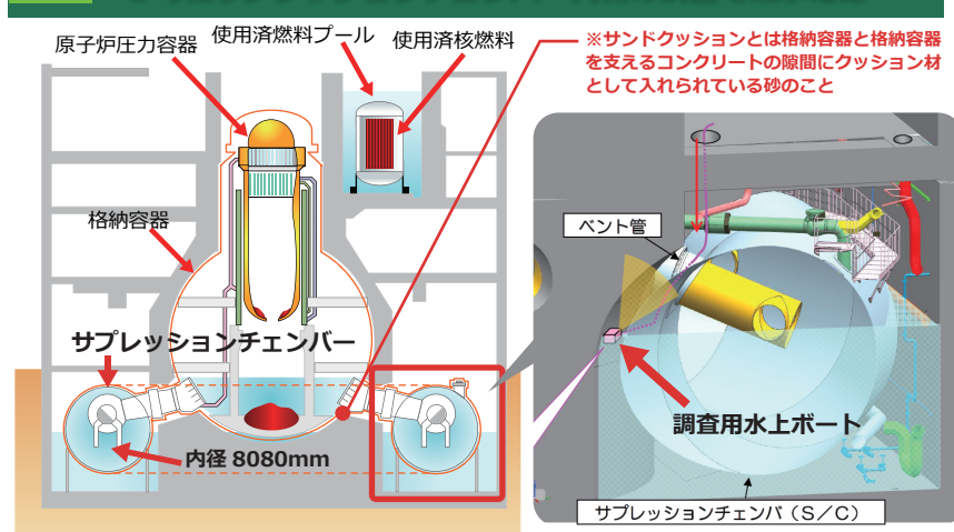
図2 1号機サブプレッションチェンバー内側の調査で漏水確認
