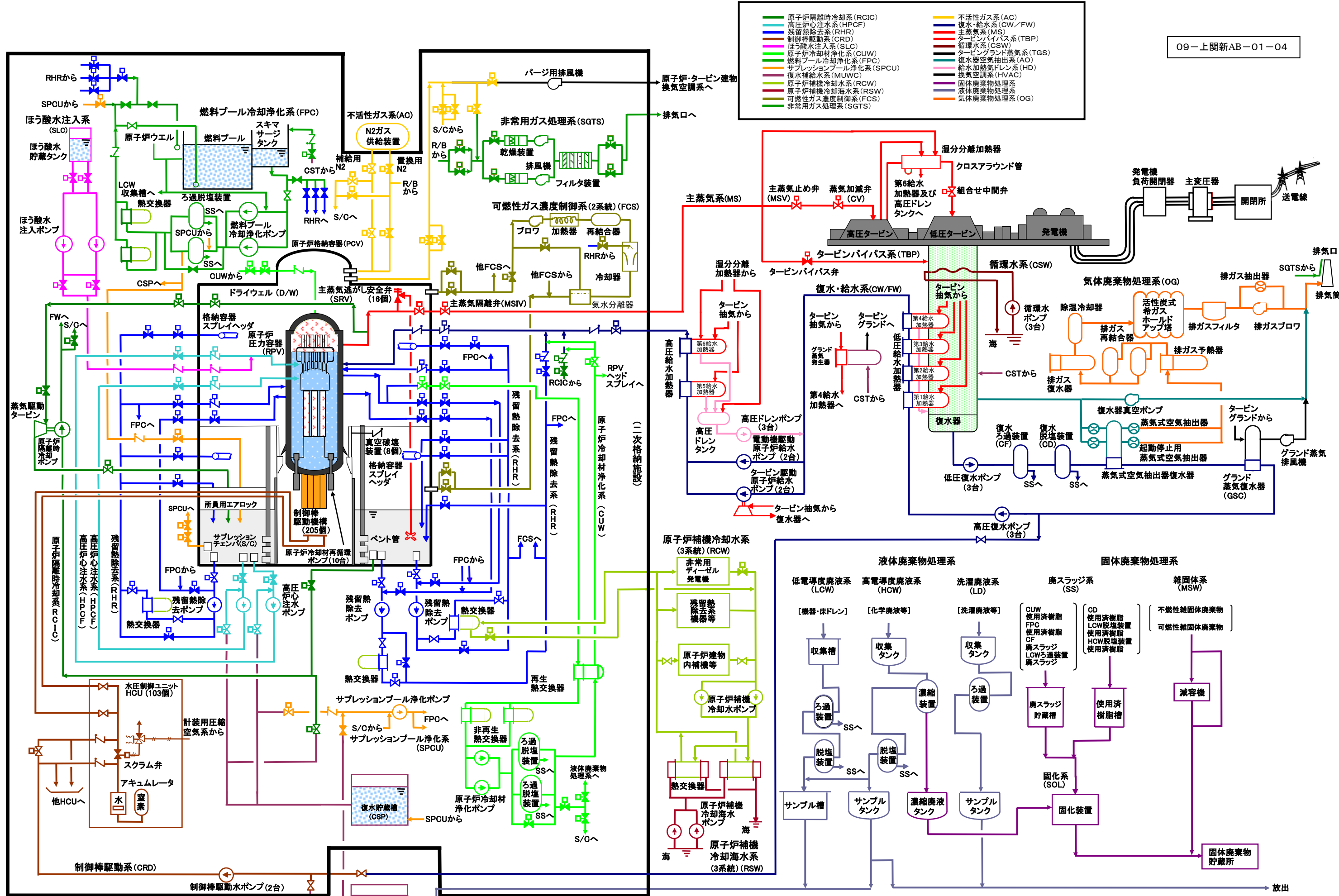
上関原子力発電所 全体系統構成概要図
